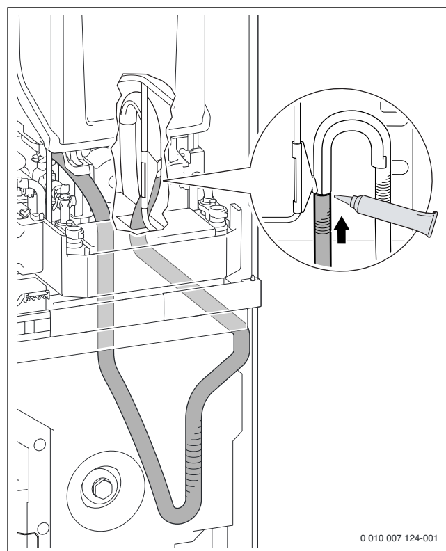
Obr. 47 Zastrčenie hadice sifónu na koncový kus
