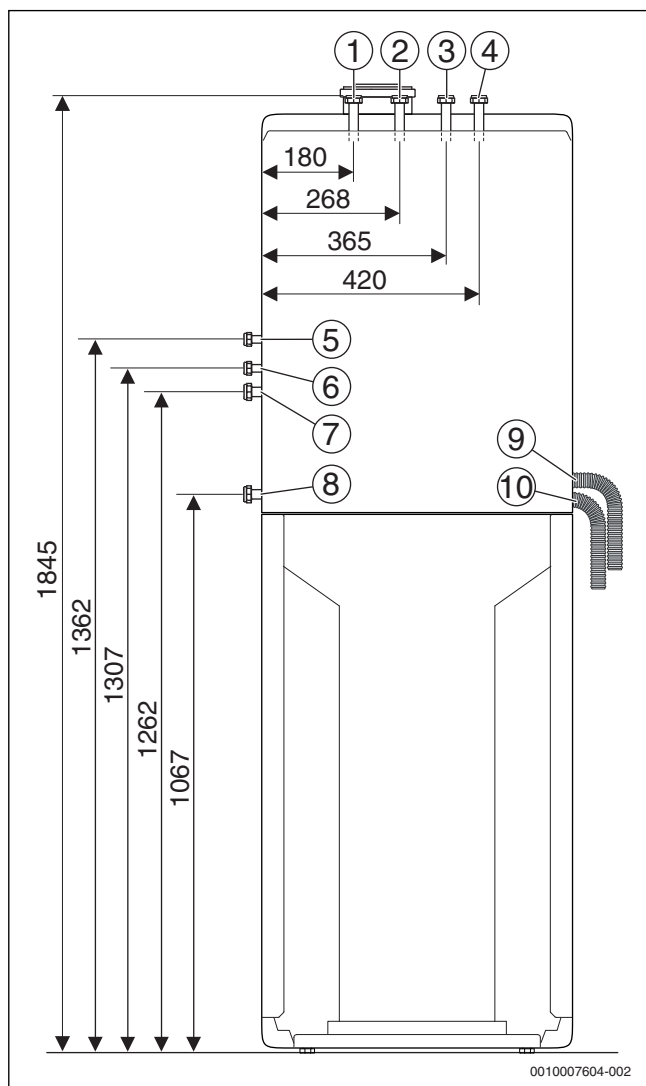
Obr. 10 Rozmery pre pripojenie príslušenstva CS13 rozšírenie vykurovacieho okruhu 2 (rozmery v mm)
