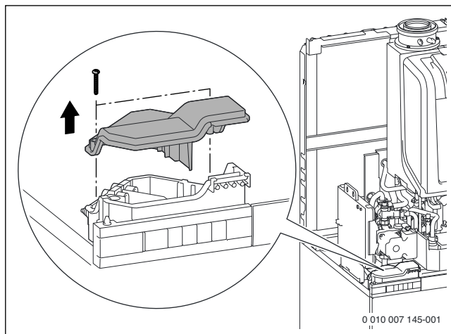
Obr. 62 Demontáž krytu pripojovacej skrine
