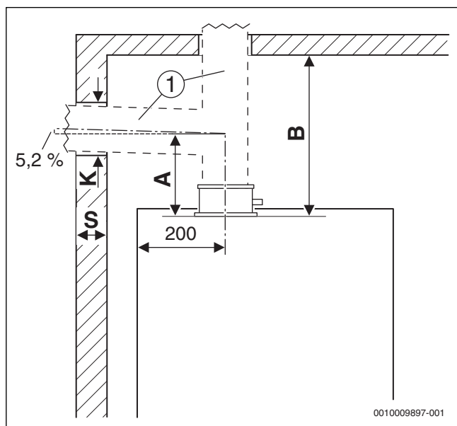
Obr. 16 Rozměry a minimální odstupy
