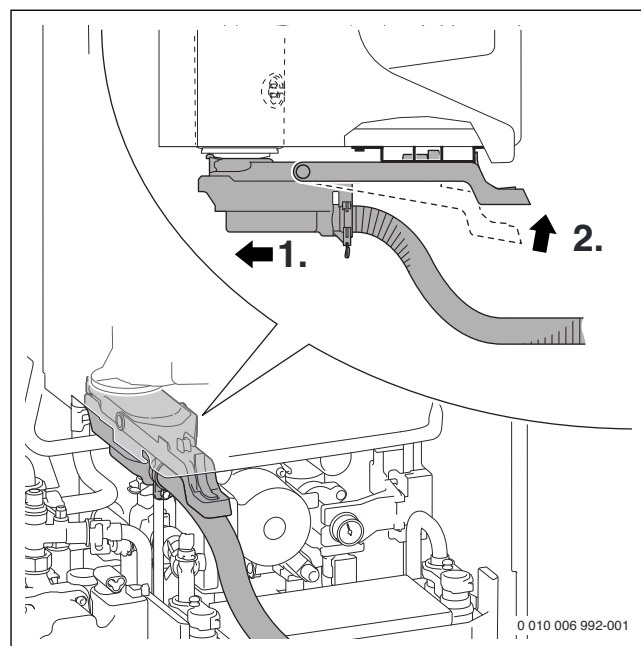
Obr. 46 Montáž filtra nečistôt
