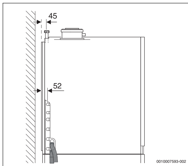
Obr. 9 Rozmery pre pripojenie príslušenstva CS12 rozšírenie vykurovacieho okruhu 1 (rozmery v mm)
