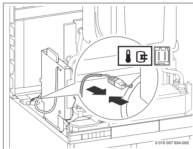
Obr. 54 Pripojenie snímača teploty zásobníka
