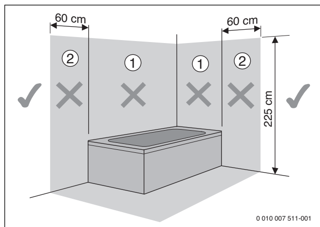
Obr. 61 Ochranné zóny
