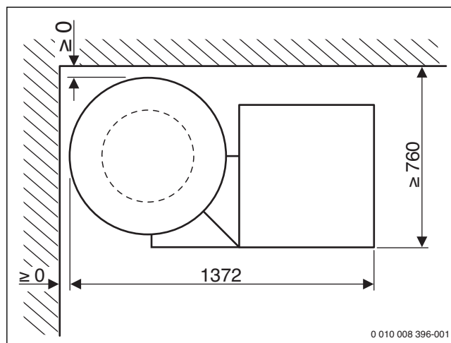
Obr. 4 Rozměry v spojení s příslušenstvom akumulacného zásobníka PNR400 (rozměry v mm)
