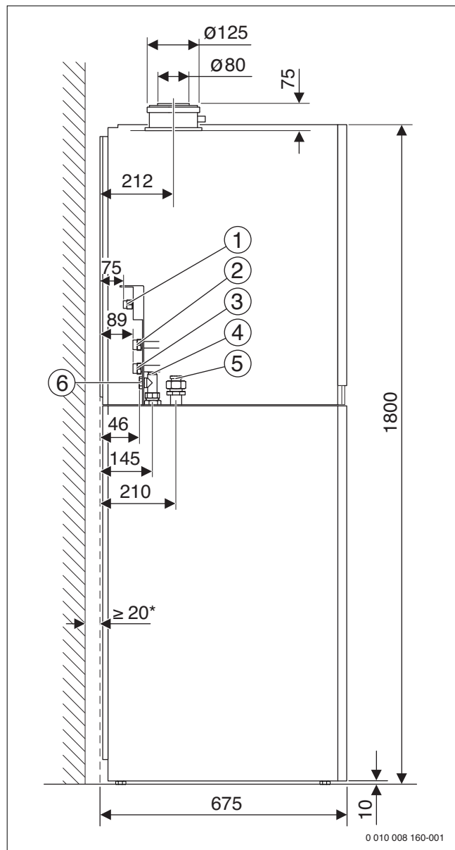
Obr. 2 Rozměry a přípojky bez příslušenstva (rozměry v mm)
