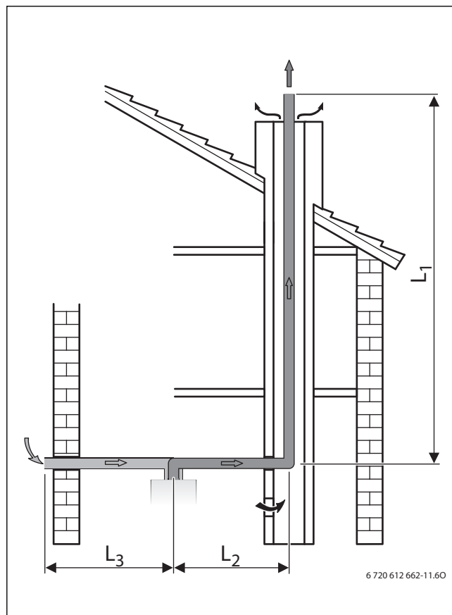
Obr. 24 Odvod spalín v šachte podľa C 53
