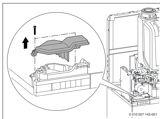
Obr. 55 Demontáž krytu pripojovacej skrine
