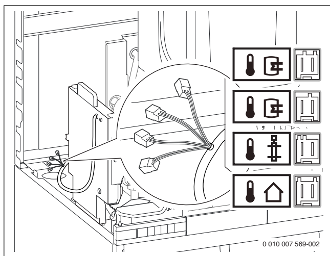
Obr. 66 Zástrčka na radiacej jednotke
