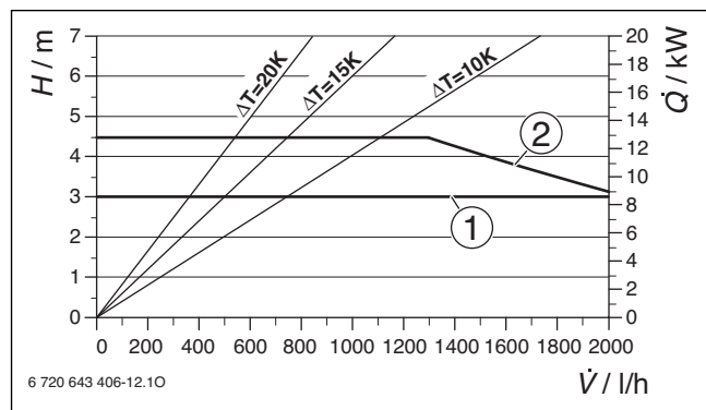
Obr. 119 Charakteristiky čerpadiel
