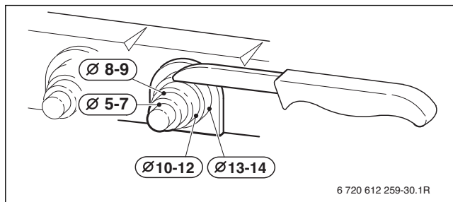
Obr. 63 Úprava spony pre odľahčenie namáhania v ťahu podľa priemeru kábla
