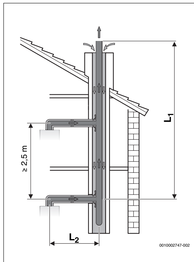
Obr. 32 Viacnásobné pripojenie pomocou koncentrickej rúry podľa C 43
