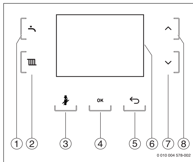
Obr. 79 Ovládací panel
