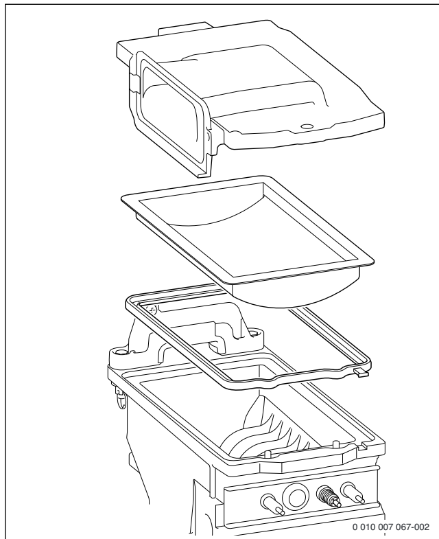
Obr. 91 Horák
