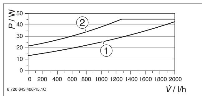
Obr. 120 Príkon
