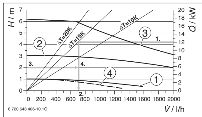
Obr. 115 Charakteristiky čerpadiel
