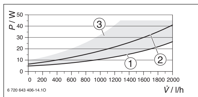
Obr. 118 Príkon
