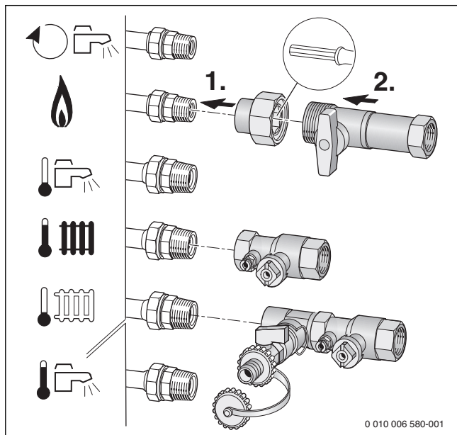
Obr. 38 Montáž sady armatúr znázornená na príklade prípojok orientovaných doprava CS10 horizontálna prípojovacia sada
