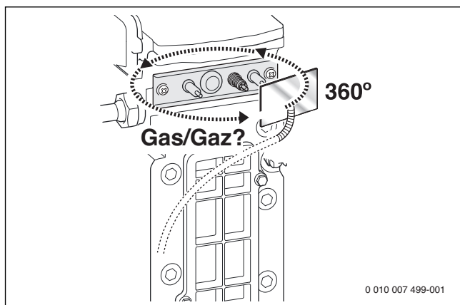
Obr. 89 Kontrola utesnenia
