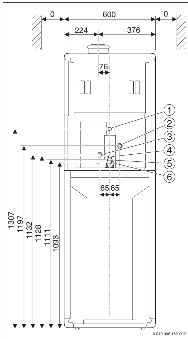
Obr. 3 Rozměry a přípojky bez příslušenstva (rozměry v mm) (odporúčaný rozmer od steny \geq 50 mm)
