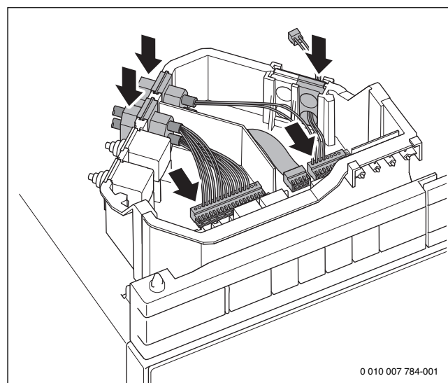
Obr. 56 Pripojenie riadiacej jednotky k pripojovacej skrini
