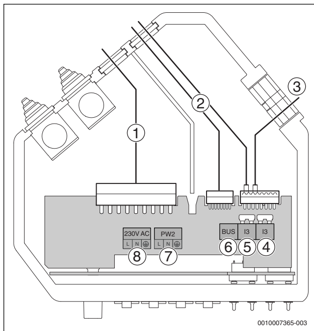
Obr. 64 Pripojovacia skriňa
