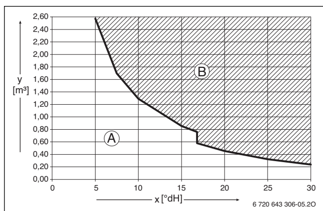
Obr. 34 Požiadavky na plniacu a doplňovaciu vodu pre kotly s výkonom < 50 kW
