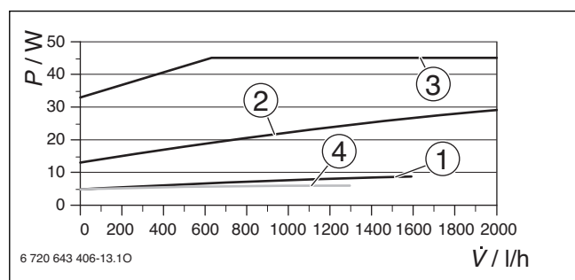
Obr. 116 Príkon
