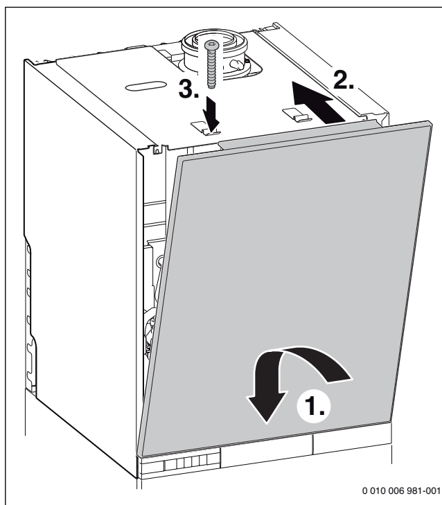
Obr. 76 Zavesenie predného krytu a jeho zaistenie dodanou skrutkou
