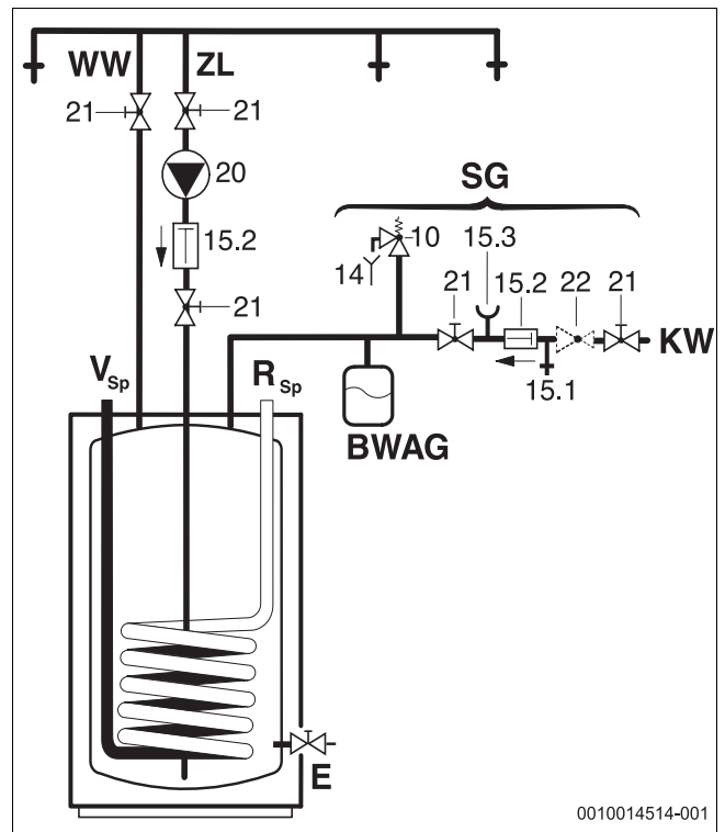
Fig. 6 Schemă de racordare la nivelul apei potabile
