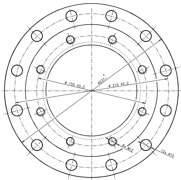
Redukčná príruha 210 / 150
